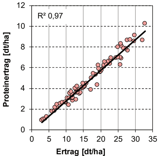
Zusammenhang von Proteinertrag und Ertrag (vom Betriebsleiter ermittelt, 86 % TS) bzw. Proteingehalt (aus Handerntproben, % i. d. TS)
