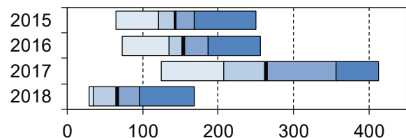
Niederschlag und Beregnung 2 Wochen nach Saat bis 3 Wochen vor Ernte [l/m²] in den 4 Untersuchungsjahren
